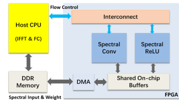
论文提出的全频段卷积神经网络的硬件加速系统
