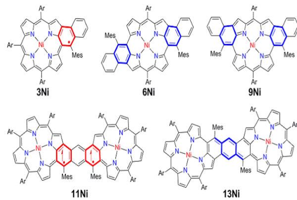
萘蒽稠合的卟啉单体和二聚体
